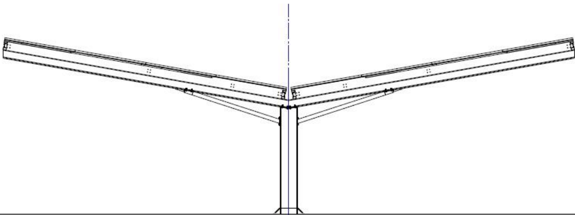
VOORAANZICHT - 1:50
